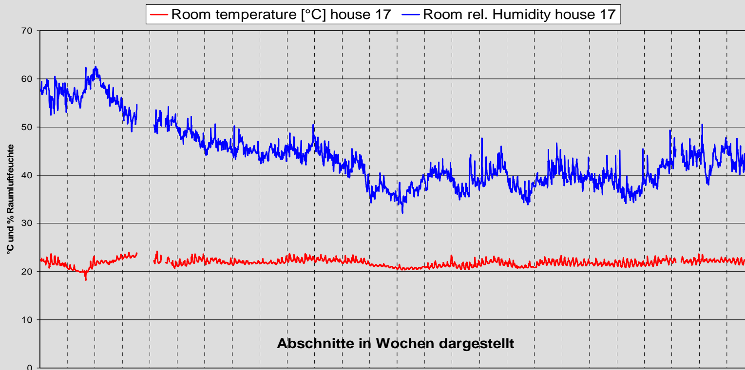
PH Wolfurt Heizperiode 2000/2001 Raumtemperaturen und rel. Raumlufffeuchte 1.10.2000 bis 31.03.2001 Zeitschritt: 60 Minuten Mittelwerte
